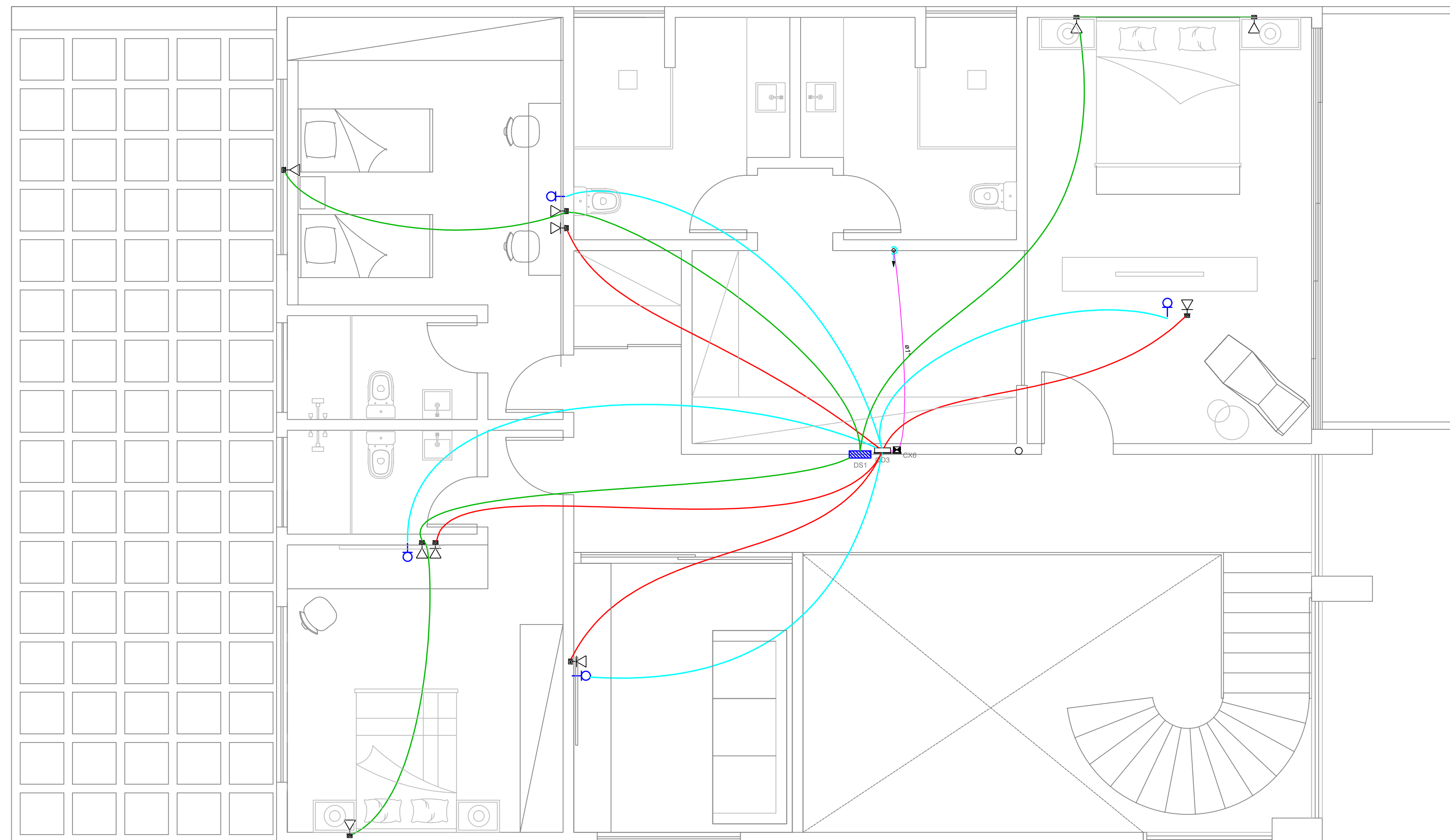
PLANTA BAIXA PAVTO. SUPERIOR - TELEFÔNICO / TV / REDE ESC. 1:50
