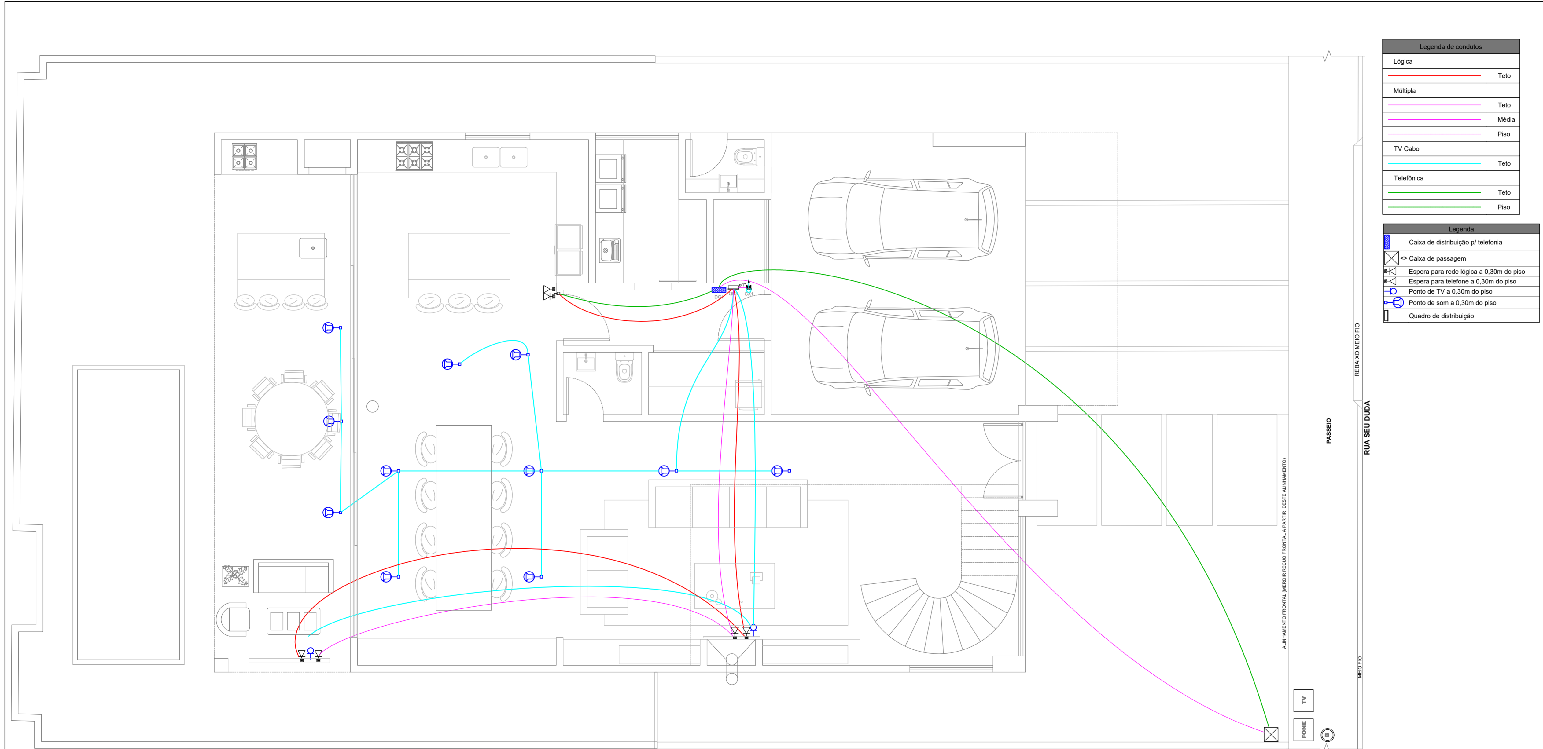
PLANTA BAIXA PAVTO. TÉRREO - TELEFÔNICO / INTERFONE / TV / REDE ESC. 1:50
