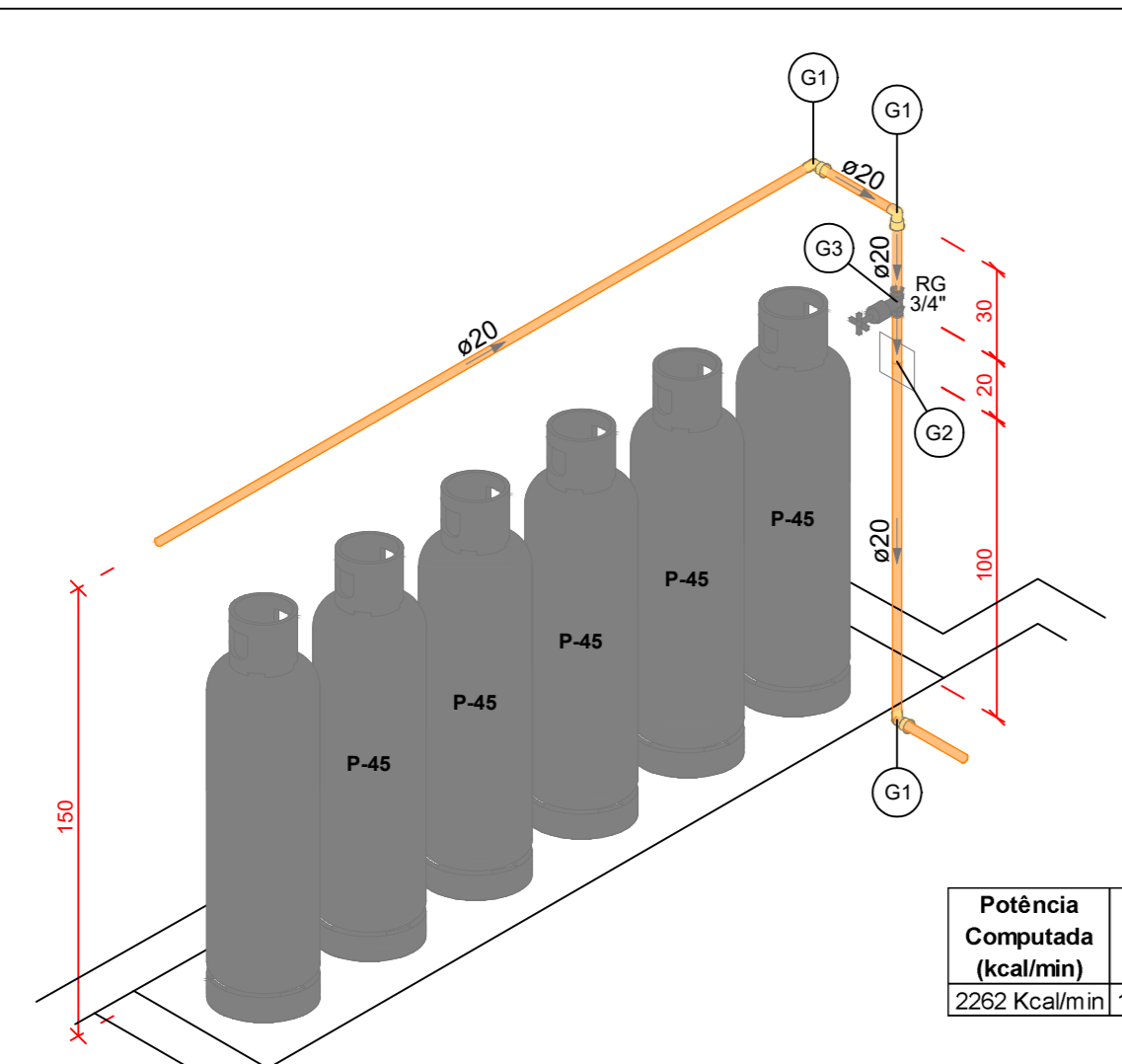
ABRIGO DE GÁS ESC.: 1/25
