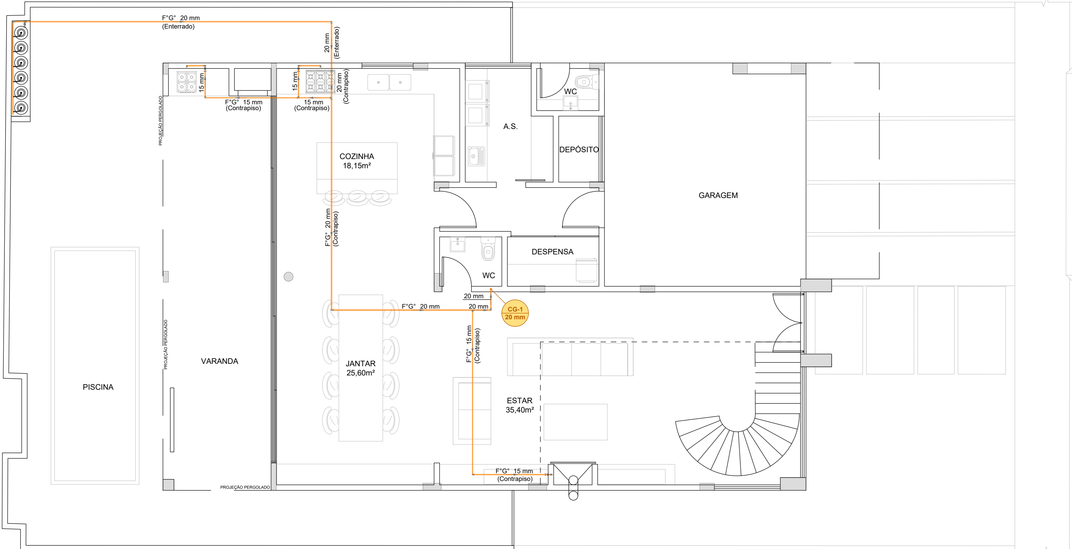
PROJETO DE GÁS - TÉRREO ESC.: 1/50
