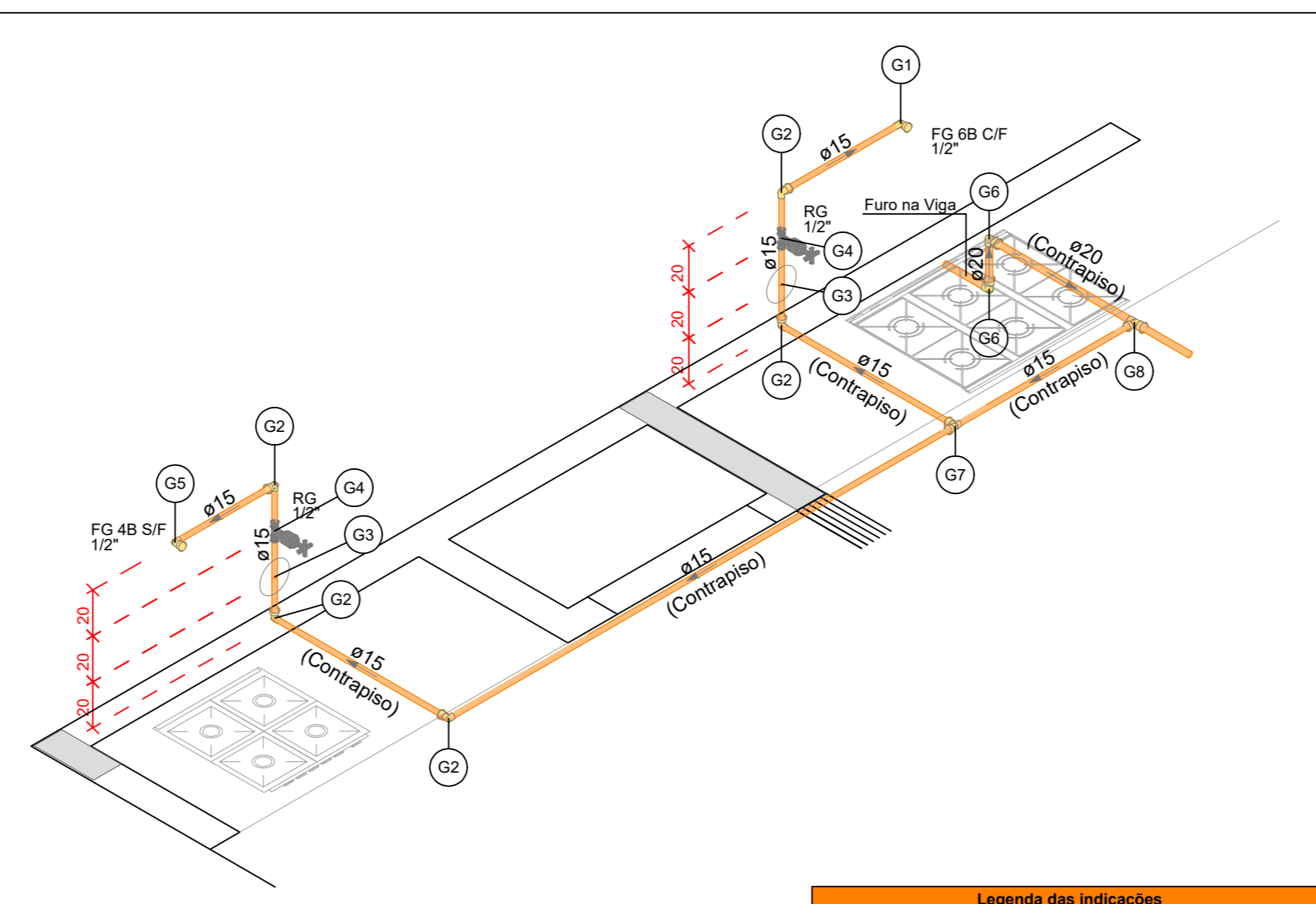
FOGÕES - TÉRREO ESC.: 1/25
