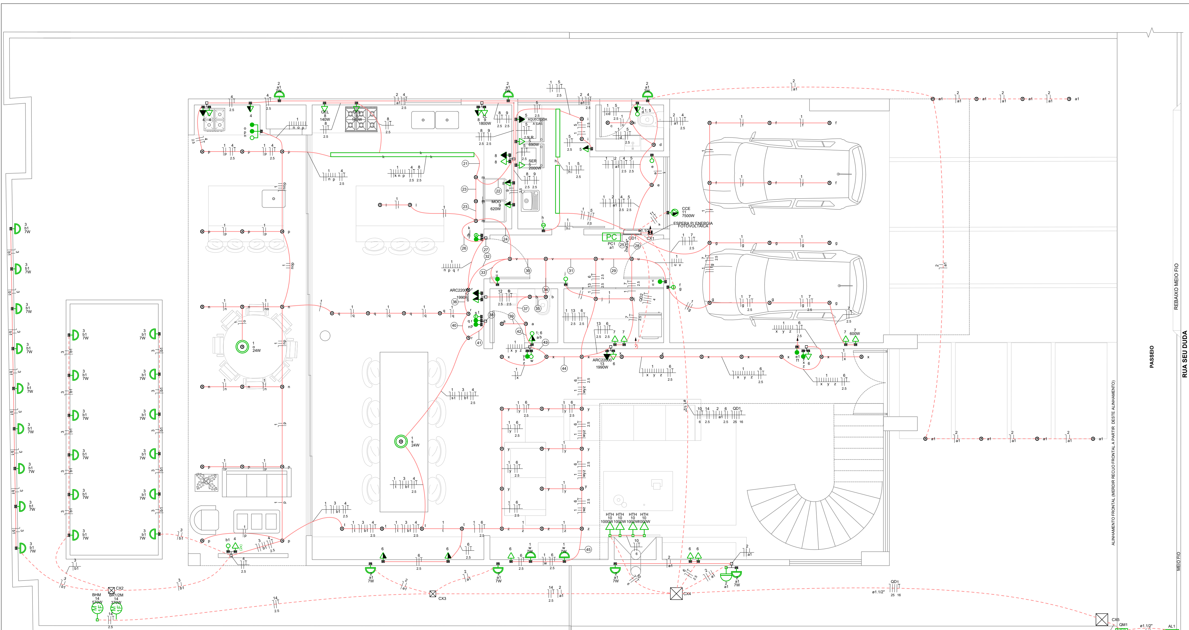
PLANTA BAIXA PAVTO. TÉRREO - INSTALAÇÕES ELÉTRICAS ESC. 1:50
